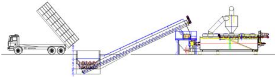
Figura 26: schema sezione impianto di ricevimento SOA. Tramoggia, trituttore primario, coclea di invio alla macinazione secondaria e cuocitore.
