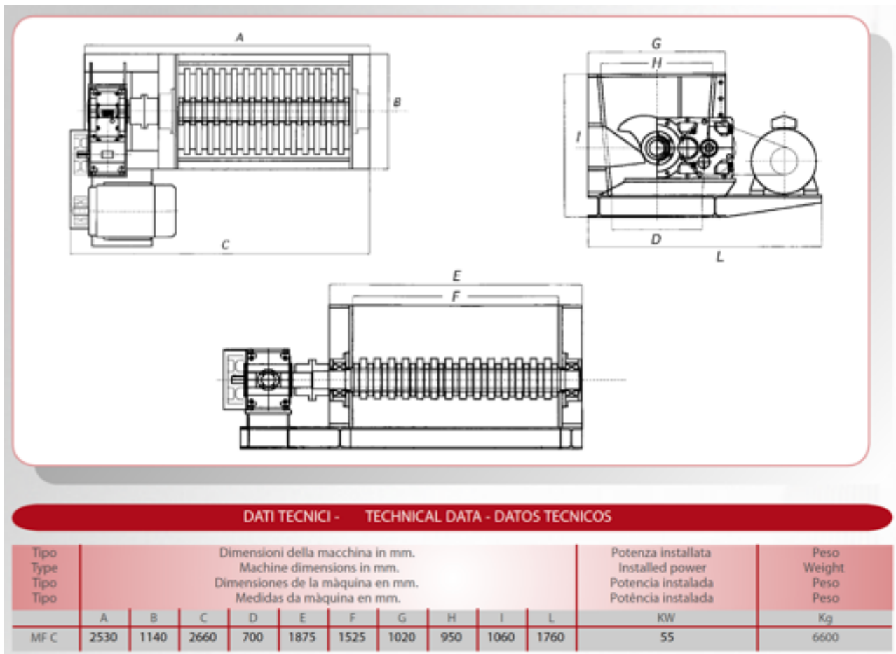
Figura 31: caratteristiche geometriche e potenza installata del trituratore primario posto nella vasca di scarico dei SOA.
