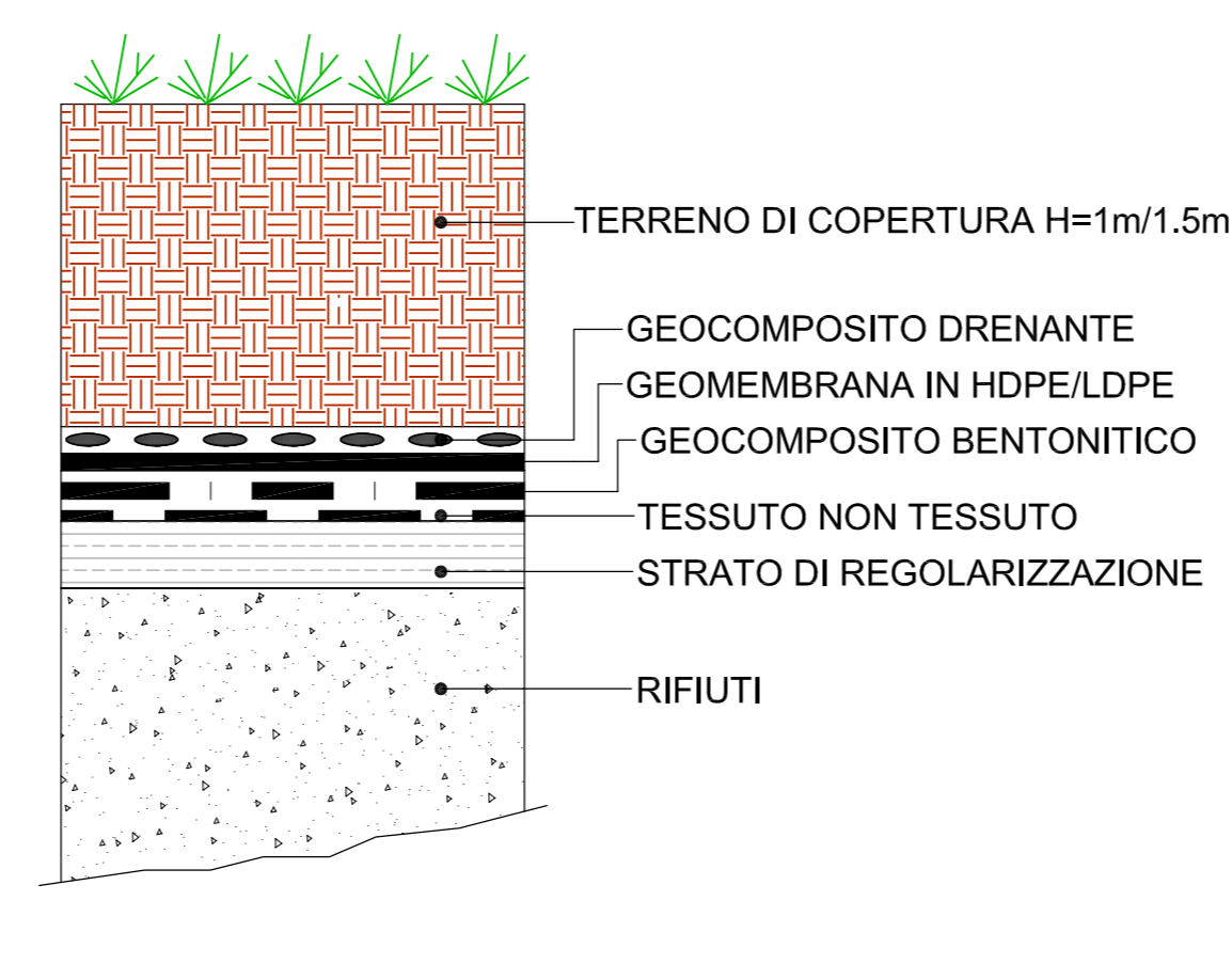
Schema di stratigrafia proposta per la ricopertura del II lotto (In ottemperanza al Dlg n°121 del 3 Settembre 2020 art. 3 2.4.3.)
