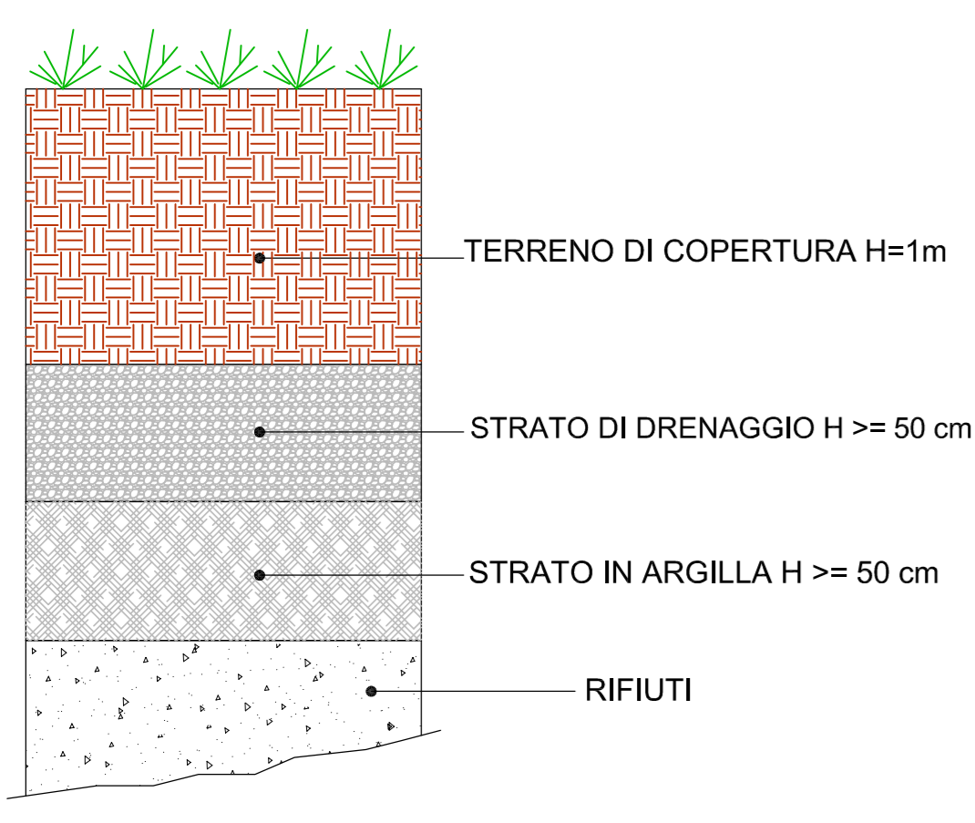
Schema di stratigrafia per la ricopertura del II lotto al Giugno 2007
