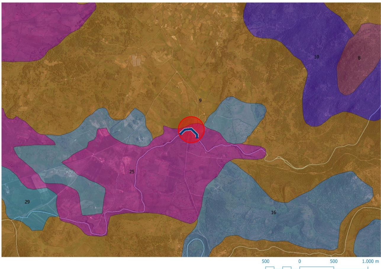
Fig.9 Carta geologica (elaborazione Multiss spa )
