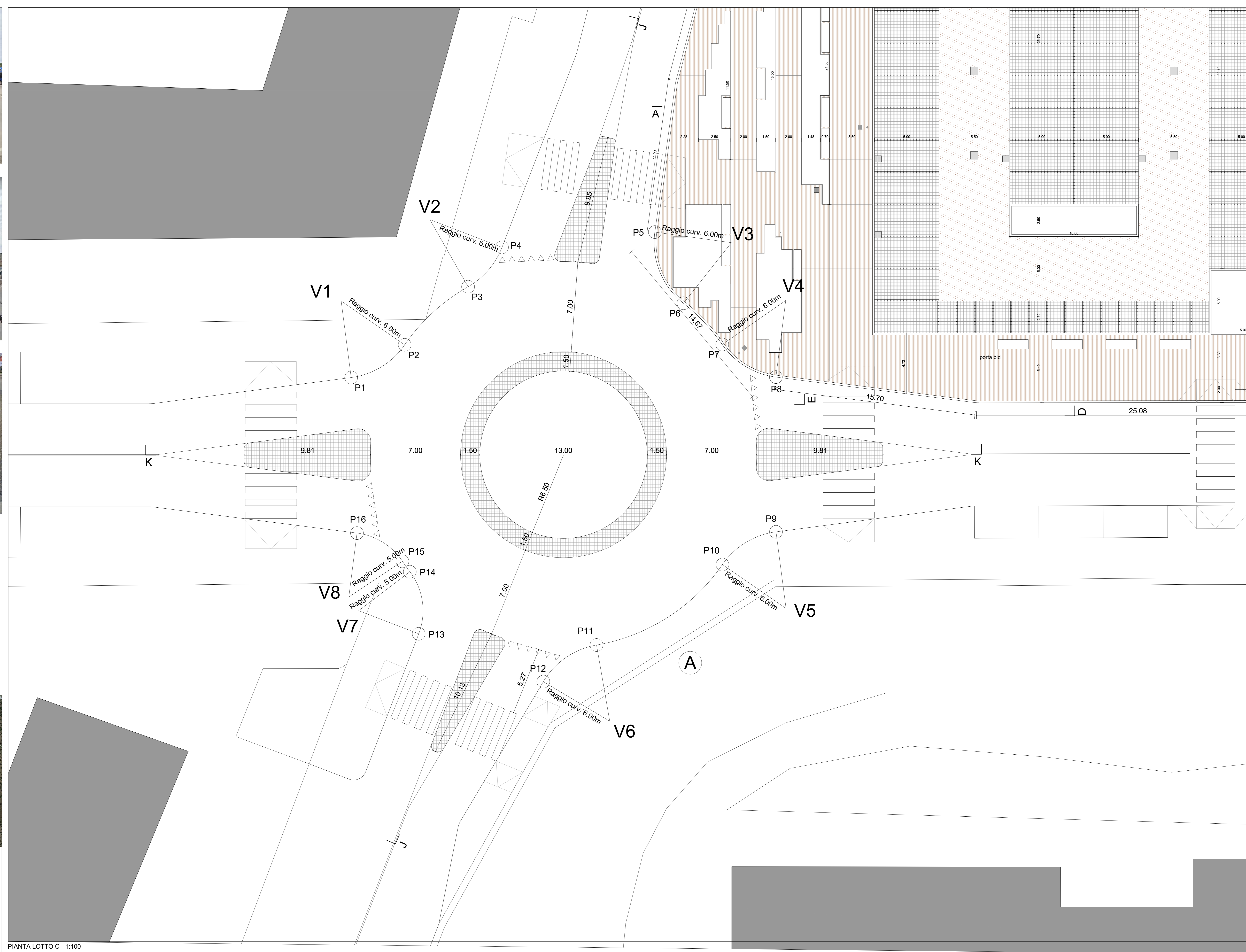
PIANTA LOTTO C - 1:100
